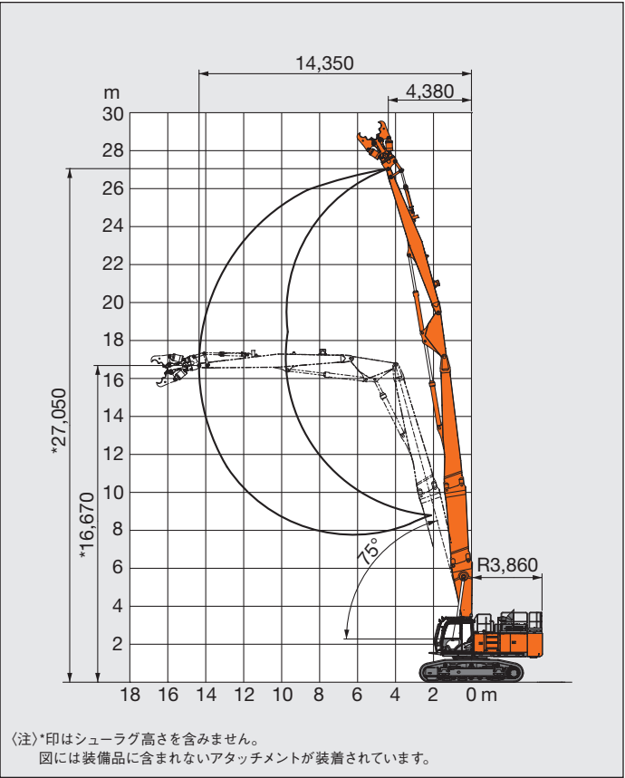
ZX480LCK-5B 27 m ハイリフトフロント仕様
