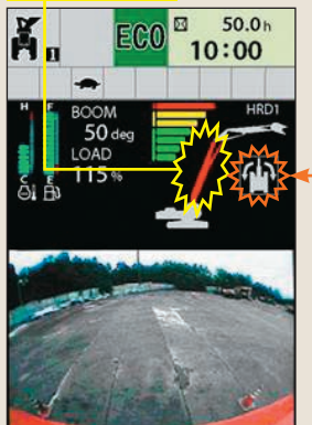
旋回角度警報
