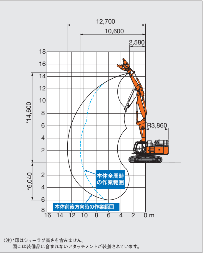
ZX480LCK-5B ツーピースブームフロント仕様
