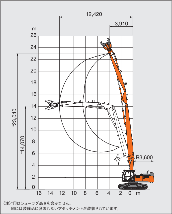
ZX350LCK-5B 23 m ハイリフトフロント仕様
