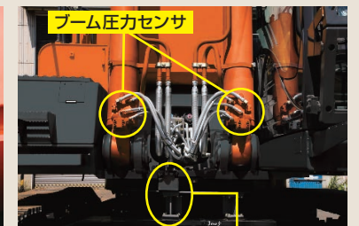
旋回角度検出装置
