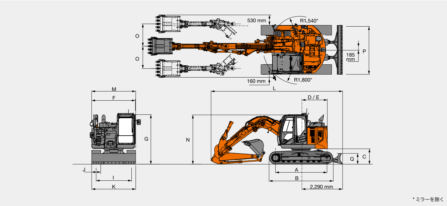
寸法図
